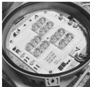
Ljusmotor (50W)
